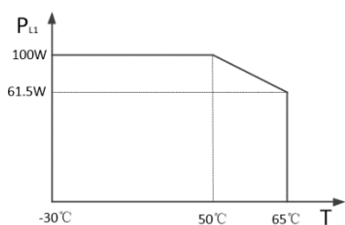
Zátěž 1 - křivka snížení výkonu Zátěž 2 - křivka snížení výkonu
