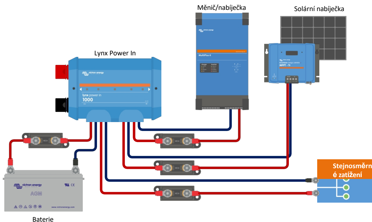
Systém pouze s přídatným zařízením Lynx Power In
