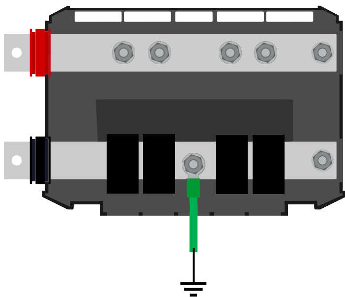
Připojení uzemnění Lynx power In
