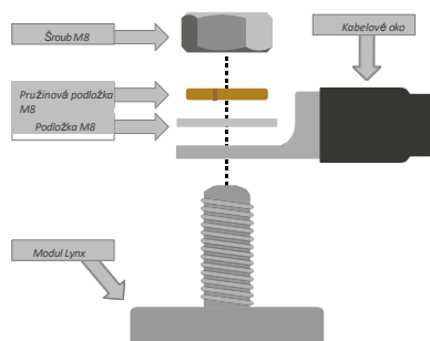
Obrázek 3. Správné pořadí montáže stejnosměrných vodičů
