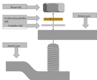
Obrázek 2. Pořadí připojení při propojení dvou modulů Lynx
