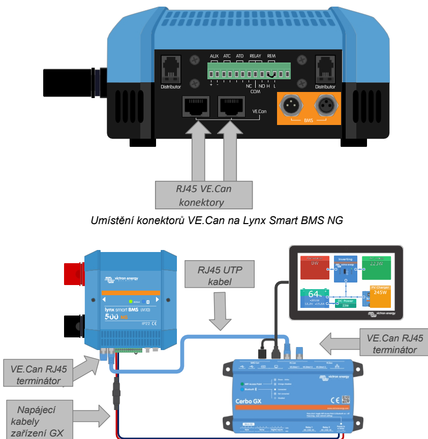
Příklad zapojení Lynx Smart BMS NG a Cerbo GX s GX Touch
