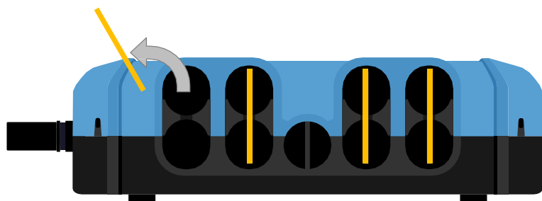
Sloupky oddělovače kabelů jsou označeny žlutě
